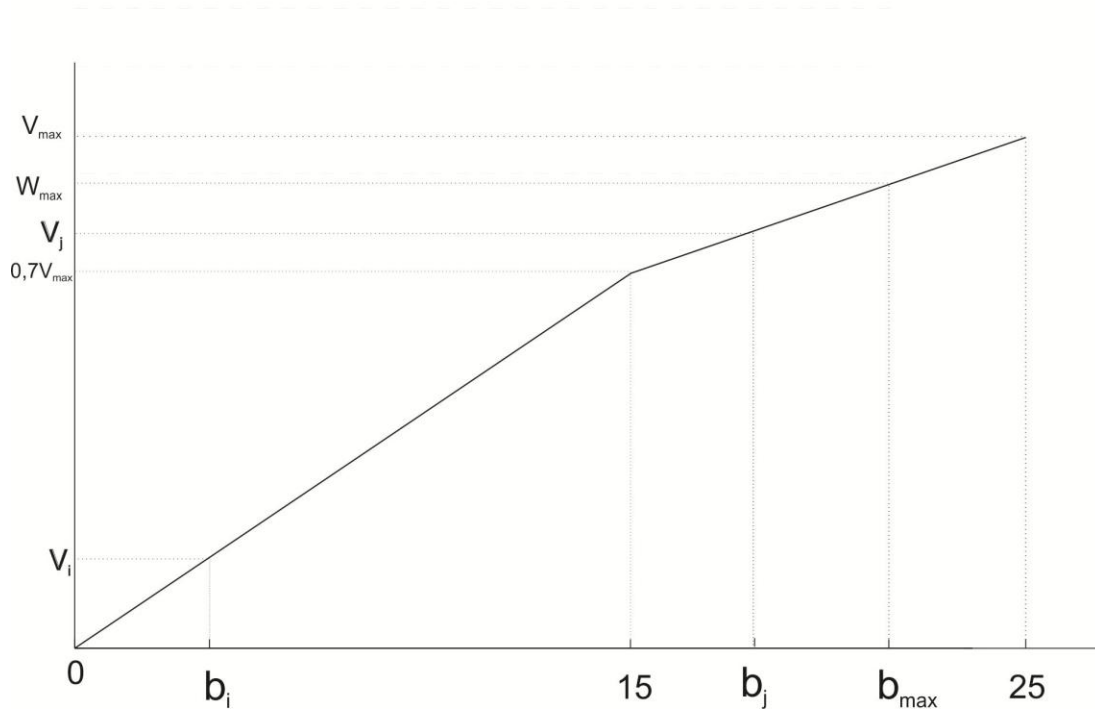
Figura 2: Representación gráfica das puntuacións se 15 \leq b_{max} < 25 .
